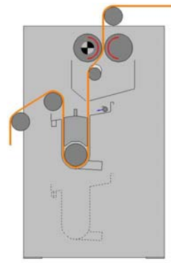
Warenlauf für Zwickelfärbung
