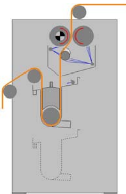
Warenlauf mit Verdränger
